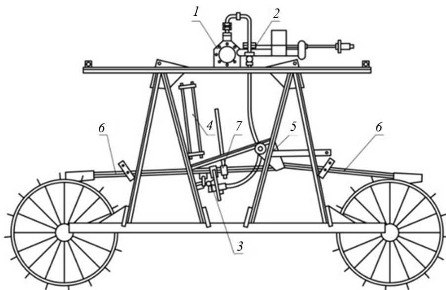
Рисунок 1 – Принципиальная схема гидравлической системы передвижения с использованием оросительной воды
