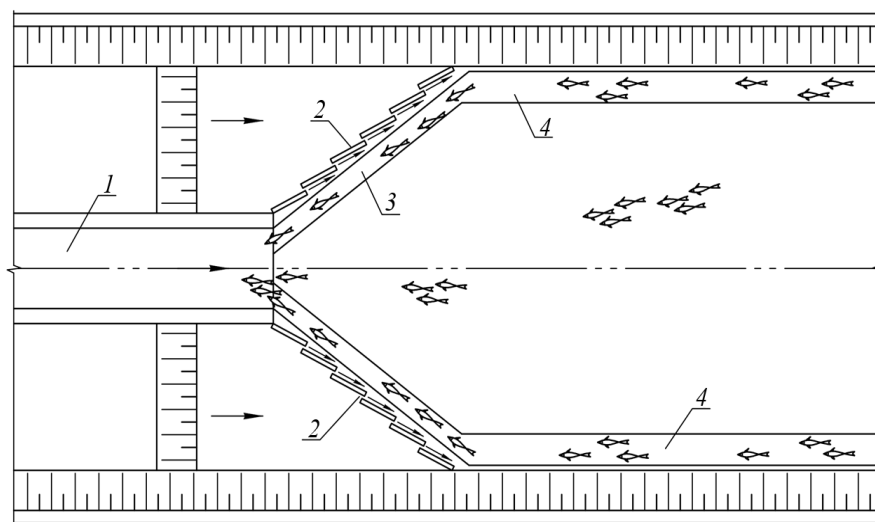
1 – рыбоаккумулятор; 2 – рыбоуправляющий порог со сквозными вертикальными щелями; 3 – рыбоуправляющая прорезь; 4 – рыбоподводящий канал
