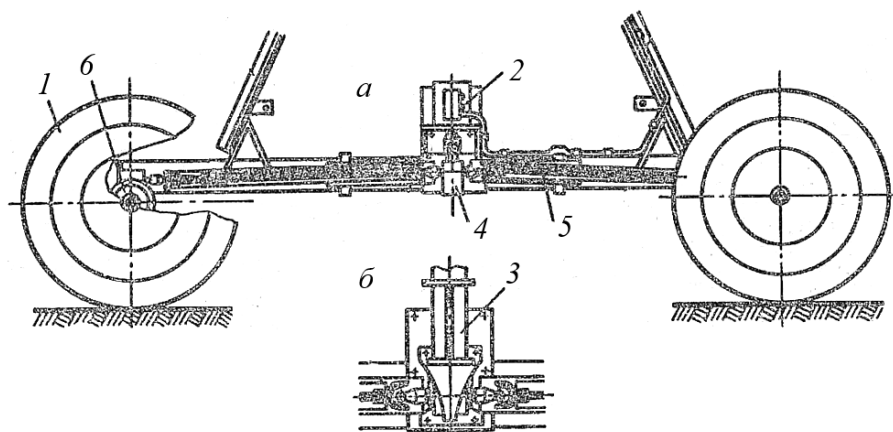
a – общий вид; б – мотор-редуктор промежуточной тележки; 1 – пневматическое колесо; 2 – электродвигатель; 3 – мотор-редуктор; 4 – червячный мотор-редуктор; 5 – трансмиссионный карданный вал; 6 – конечный червячный редуктор
