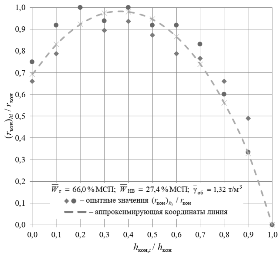
Рисунок 3 – Примеры функциональной связи (r_{kon})_{h_i} / r_{kon} = \int \cdot (h_{kon,j} / h_{kon})
