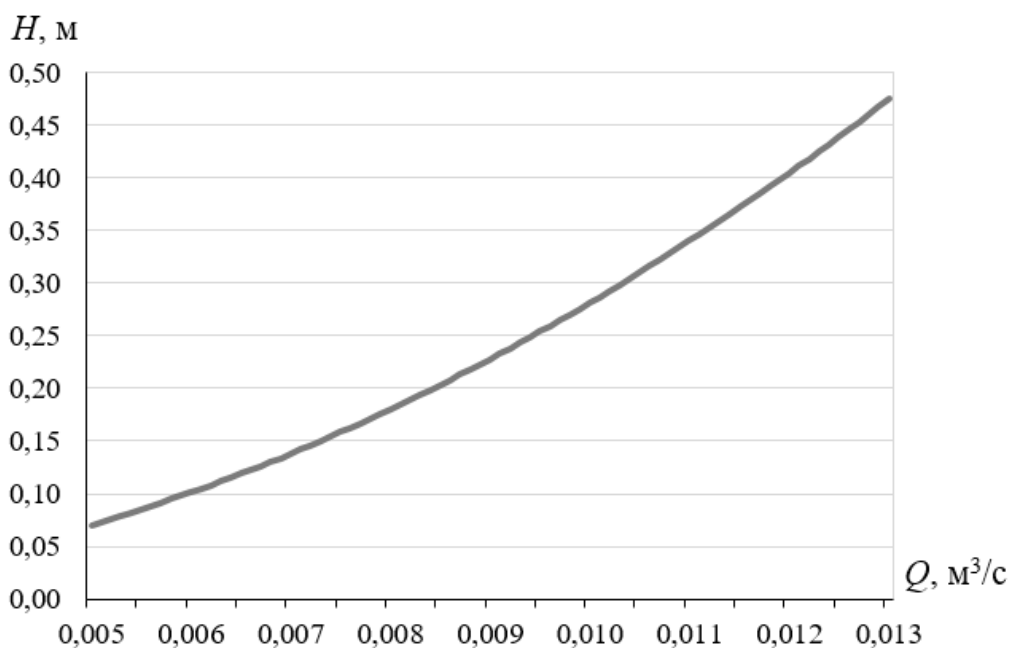
Рисунок 6 – Кривая Q = f(H) лабораторного образца регулятора уровня
