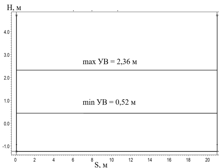
Рисунок 5 – Поперечное сечение русла реки в створе ИК 239
