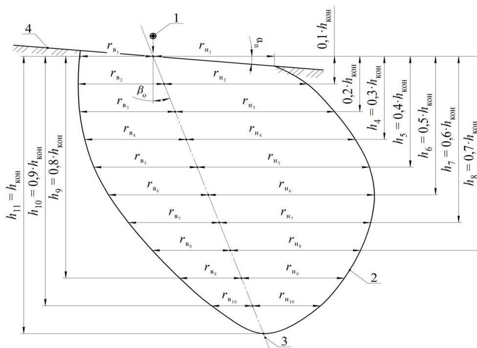
Рисунок 5 – Схема контура влажности, формирующегося на склоновых землях
