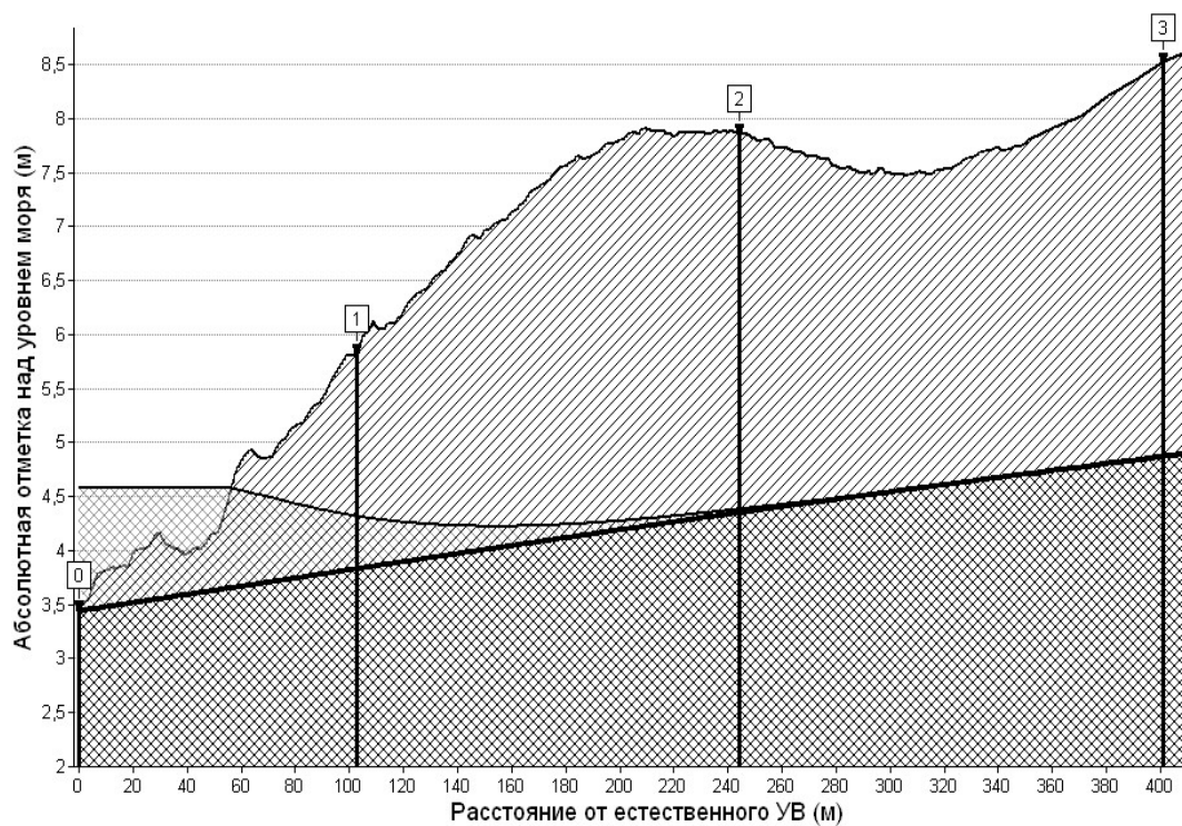
Рисунок 4 – Пример графика, отображающего изменение уровня грунтовых вод в створе при поднятии уровня воды в водном объекте
