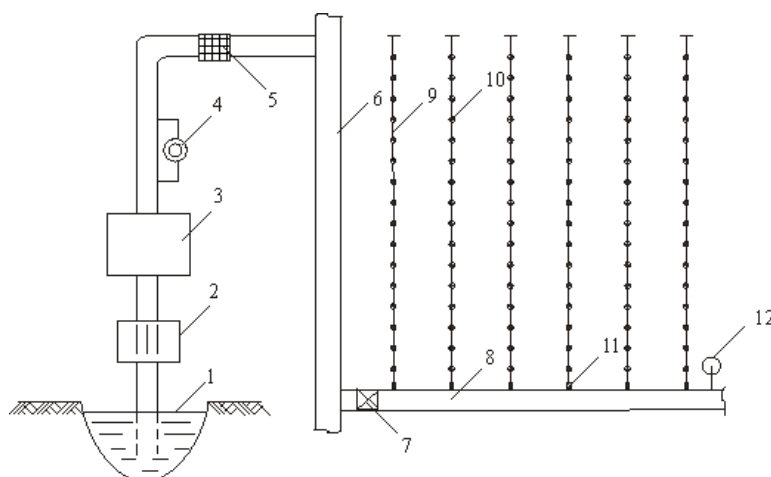
Рисунок 1 – Условная схема системы комбинированного орошения
