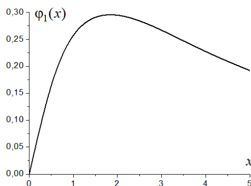
Рисунок 2 – График функции \varphi_1(x)
