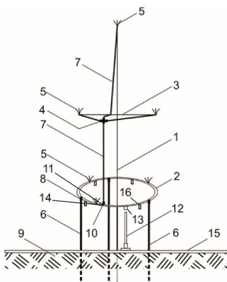
Рисунок 2 – Аэрозольная установка для увлажнения плодовых насаждений
