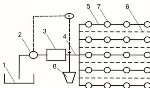
1 – водоисточник; 2 – насосная станция; 3 – блок фильтров; 4 – распределительный трубопровод; 5 – комбинированный трубопровод; 6 – разделительная полоса; 7 – комбинированные установки; 8 – емкость H_2O + O_2 ; К – контроллер
