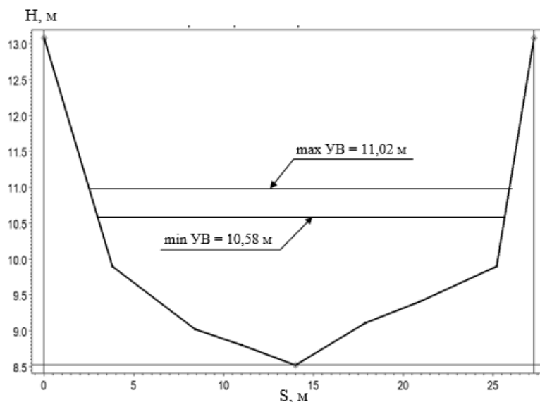
Рисунок 4 – Поперечное сечение русла реки в створе ИК 241
