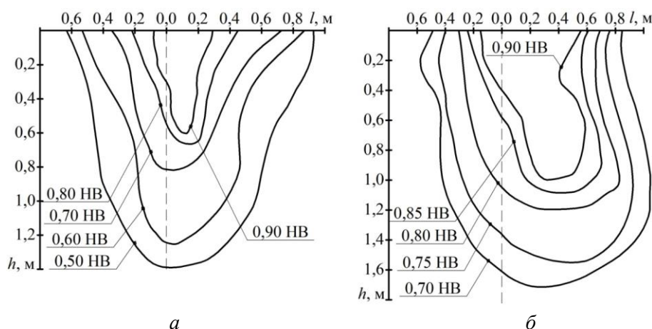
Рисунок 3 – Контурсы влажности почвы, формирующиеся на склоновых землях при капельном поливе, по И. К. Кулиничу [7]
