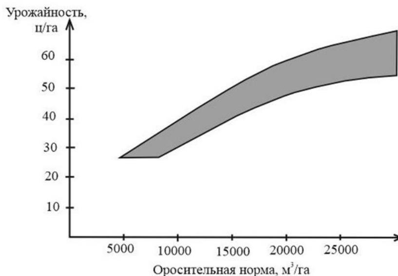
Рисунок 1 – Область значений производственных функций для риса, возделываемого на землях Черноерковской оросительной рисовой системы
