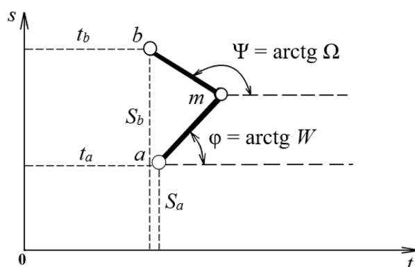
Рисунок 1 – Графический анализ системы по формуле (4)
