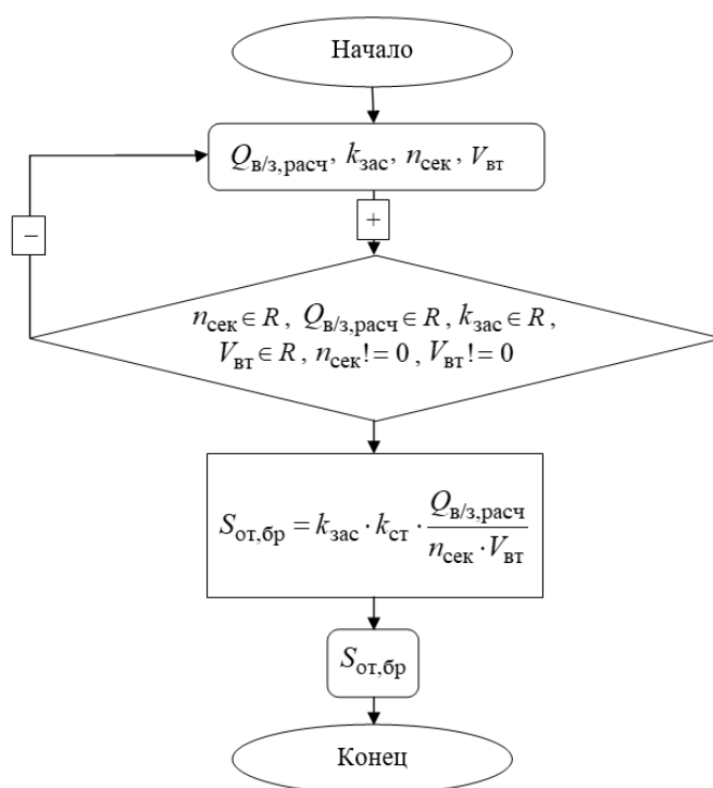
Рисунок 1 – Блок-схема алгоритма вычисления расчетной площади водоприемного отверстия брутто, m^2
