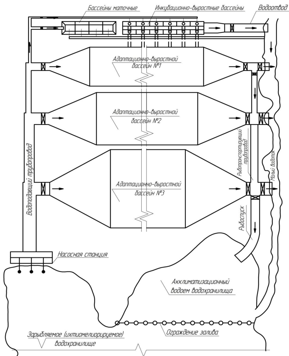
Рисунок 1 – Компоновочная схема приводохранилищного рыбоводно-мелиоративного комплекса
