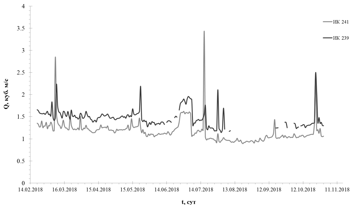
Рисунок 2 – Динамика расходов воды р. Темерник по результатам измерений ИК 241 и ИК 239 в 2018 г. на 0 ч
