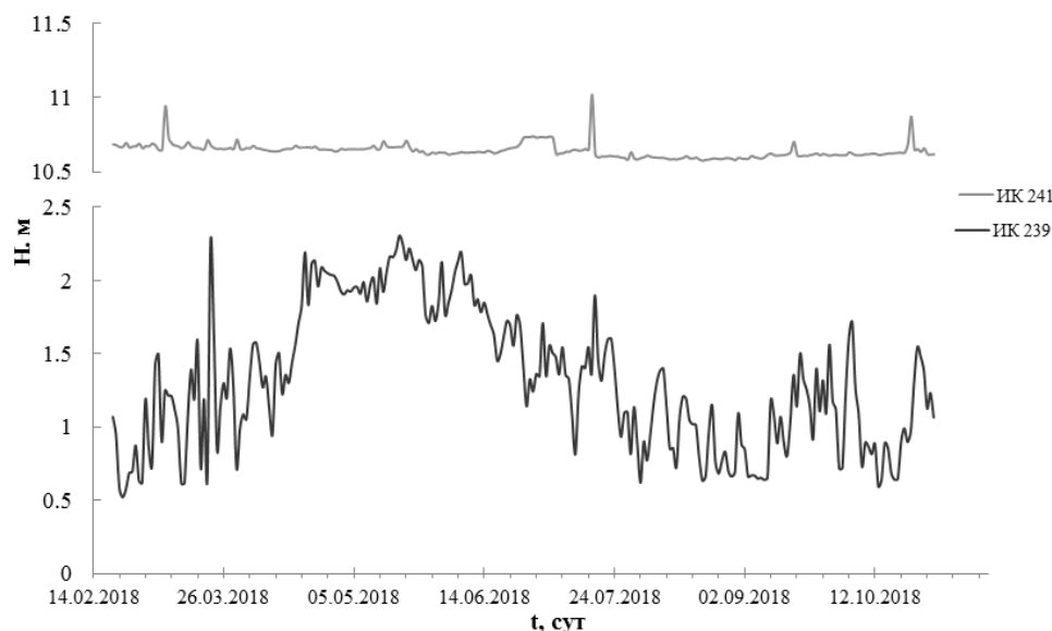
Рисунок 3 – Динамика уровней воды р. Темерник по результатам измерений ИК 241 и ИК 239 в 2018 г. на 0 ч
